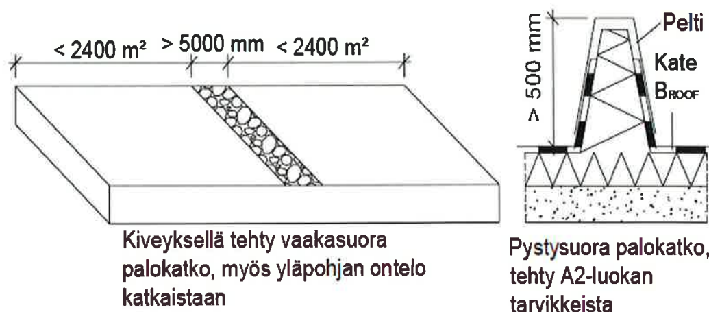
Kuva 1. Palokatkojen periaatteet Ympäristöopas 39:n mukaan [A4].
